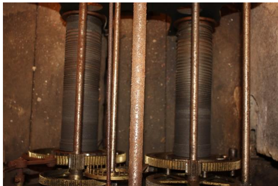
Figura 25 - Pormenor da máquina do relógio
